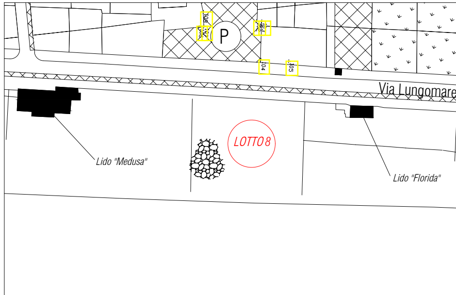
PLANIMETRIA LOTTO 8 - SCALA 1:2000
